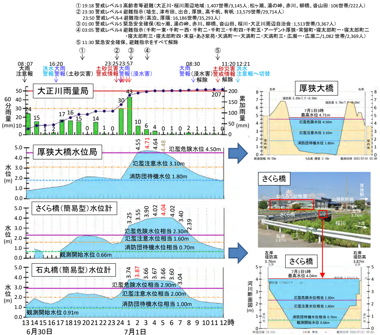
図 11 大正川雨量局、厚狭大橋・さくら橋（簡易型）・石丸橋（簡易型）水位局における雨量・水位の推移、厚狭大橋・さくら橋の断面図、さくら橋簡易型水位計の設置状況（山口県土木防災情報システムより転載・加筆、写真は筆者らが撮影）
