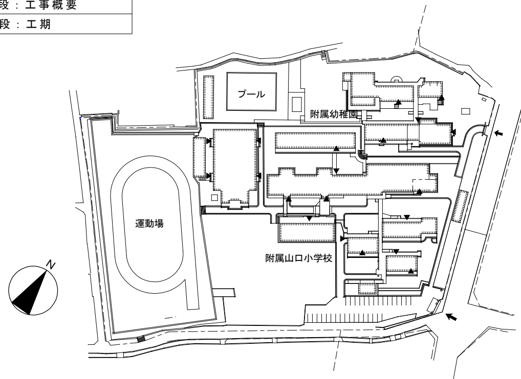
白石3丁目団地配置図
