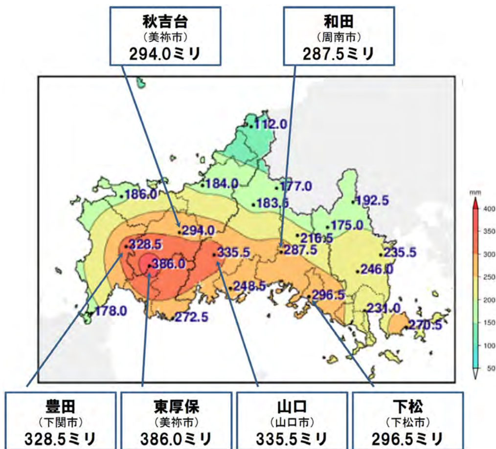
図4 アメダス総降水量の分布図（6月29日～7月1日、3日間、72時間）（下関地方気象台、2023）
