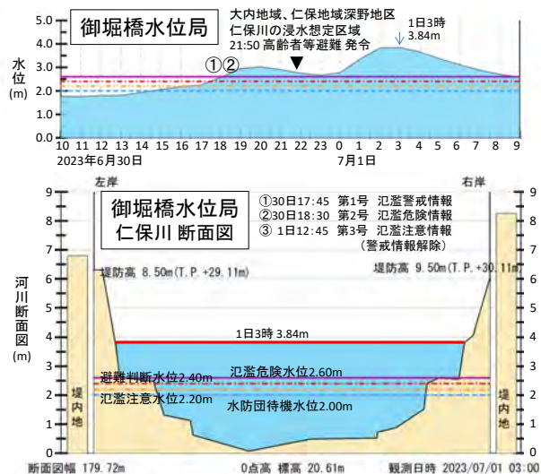
図7 2023年6月30日10時から7月1日9時までの鰐石雨量局、朝田・大歳・九田・御堀橋の水位局における雨量・水位、防災情報の推移、榎野川・吉敷川・九田川・仁保川の断面図
