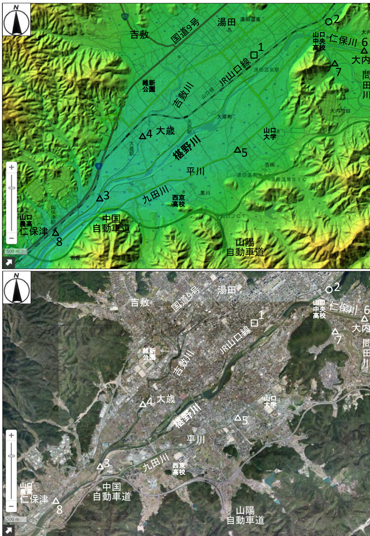
図6 山口市の平川・大歳・大内・仁保津地域の色別標高図（上）と空中写真（下） （国土地理院「地理院地図」より転載・加筆）（図中の口は1：山口アメダス、○は雨量局 （2：鰐石雨量局）、△は水位局（3：朝田水位局、4：大歳水位局、5：九田水位局、 6：御堀橋水位局、7：姫山橋簡易型雨量計、8：茶屋川簡易型水位計）
