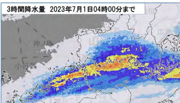
図2 3時間降水量の解析雨量（6月30日23時から7月1日04時までの1時間毎） （下関地方気象台、2023）
