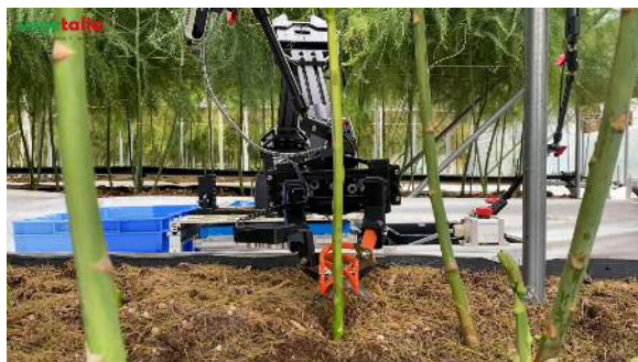
アスパラ収穫ロボット
